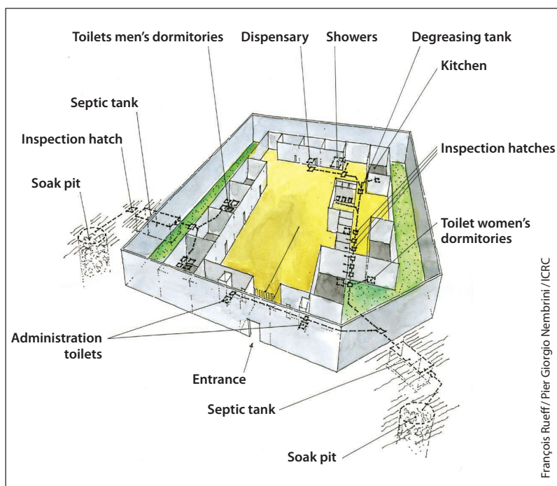
รูป 19 ระบบรวบรวมและระบายน้ำเสีย องค์ประกอบของระบบส่วนใหญ่ฝังอยู่ใต้ดิน
