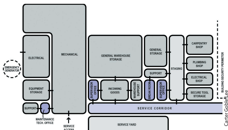
รูป 12 การปฏิบัติการและการบำรุงรักษา (แผนภูมิขอบเขต โครงสร้างพื้นฐาน ที่จำเป็นต้องมี)
