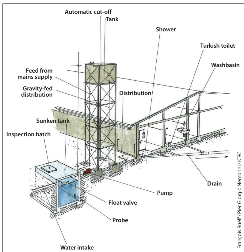
รูป 17 ระบบน้ำตามแบบฉบับที่มีบ่อเก็บน้ำใต้ดินและถังเก็บน้ำยกระดับเพื่อให้แน่ใจว่ามีความดันเหมาะสมพอที่จะจ่ายน้ำผ่านท่อไปยังสิ่งอำนวยความสะดวกต่าง ๆ และที่สำคัญคือการผลักดันน้ำเสียทิ้ง
