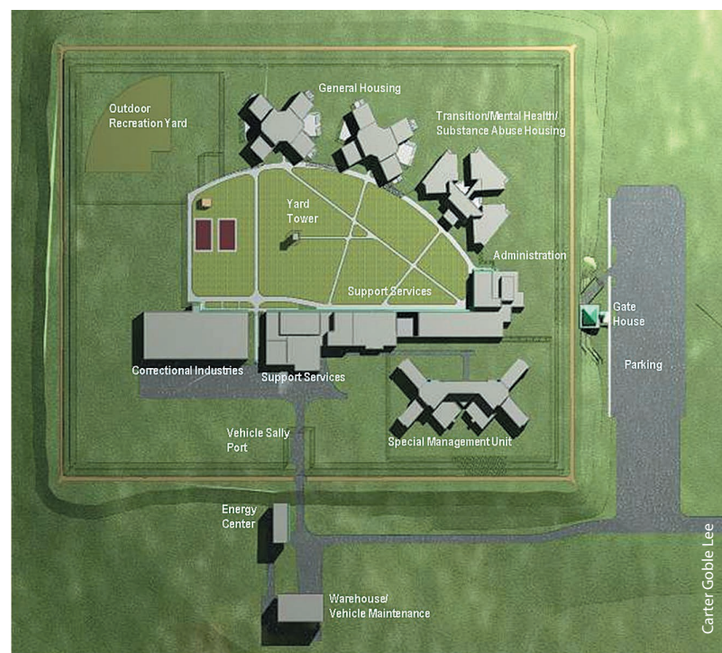
รูป 1 ตัวอย่างบริเวณเรือนจำที่มีสิ่งอำนวยความสะดวกและบริการขั้นพื้นฐาน
